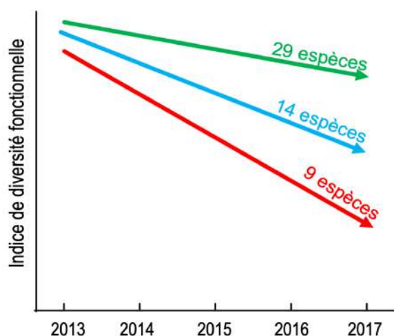
Figure 4. Évolution de la diversité fonctionnelle des plantes selon le nombre d'espèces semées au départ. Les mélanges restent d'autant plus stables qu'ils ont été semés avec beaucoup d'espèces. Résultat d'un essai à Grignon (Yvelines).
