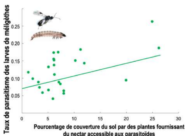
Figure 3. Le pourcentage de couverture du sol en avril par des plantes en fleur fournissant du nectar aux parasitoïdes augmente le taux de parasitisme des melligèthes du colza. Résultat d'un essai en parcelle expérimentale à Grignon (Yvelines).
