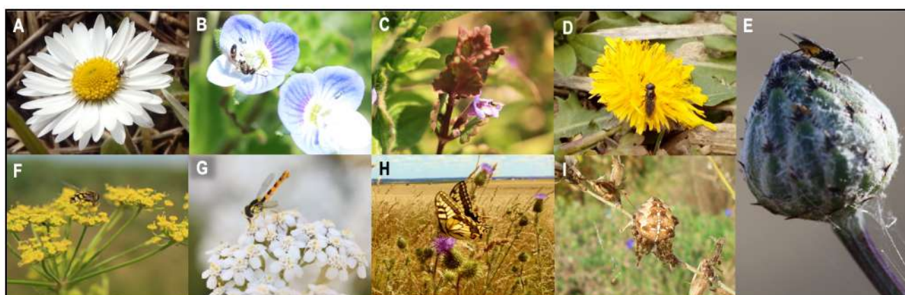
Figure 1. Les plantes à floraison précoce comme la pâquerette (A), la véronique de Perse (B), le gléchoïde faux-lierre (C) et le pissenlit (D) nourrissent les parasitoïdes d'altises et de méligèthes (A, B et C) ainsi que les syrphes (D) dès le mois de février. Le nectar peut aussi être produit en été sur le bouton floral, comme chez la centaurée scabieuse (E). Les fleurs à corolle ouverte comme chez la véronique (B) et le panais (F), ou à nectar peu profond comme chez l'achillée (G) offrent du nectar aux syrphes ayant des langues courtes. D'autres fleurs non semées favorisent la biodiversité, autre que les auxiliaires, comme le machaon (H). Les bandes fleuries sont enfin des habitats stables pour les prédateurs comme les carabes et les araignées (I).
